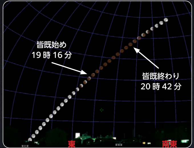
図：11月8日の月の軌道、16時10分から10分おきに表示
